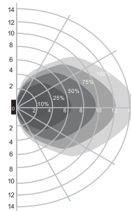
Wall mounting pattern (Unit: m) Suggested installation height: 1-1.8m Patrón de montaje en pared (Unidad: m) Altura de instalación sugerida: 1-1.8m
