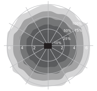
Ceiling mounting pattern (Unit: m) Suggested installation height: 2.5-6m Gráfica de montaje de techo (Unidad: m) Altura de instalación recomendada: 2.5-6m
